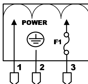
POWER MODULE
